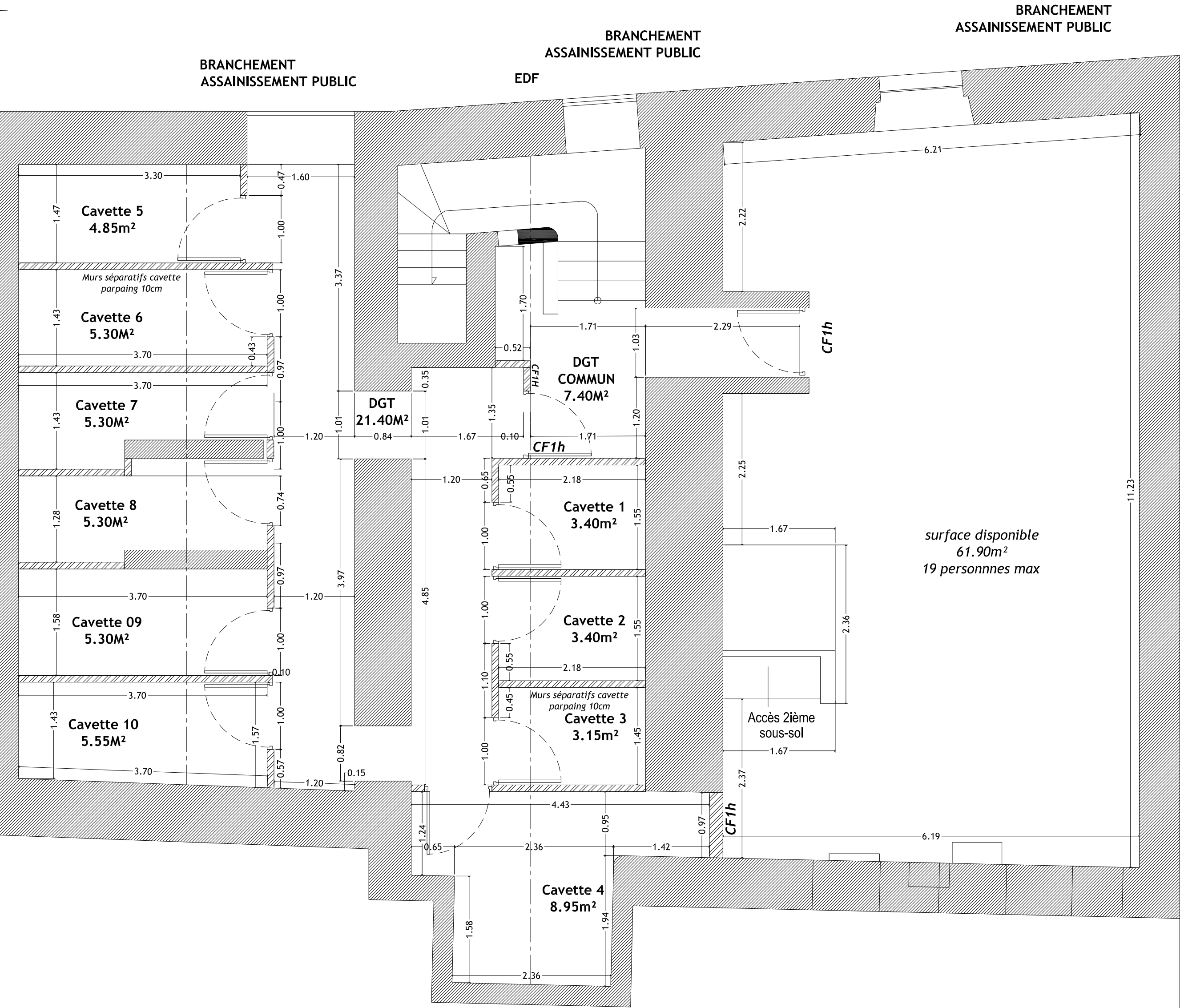
PLAN R-1 PROJET
