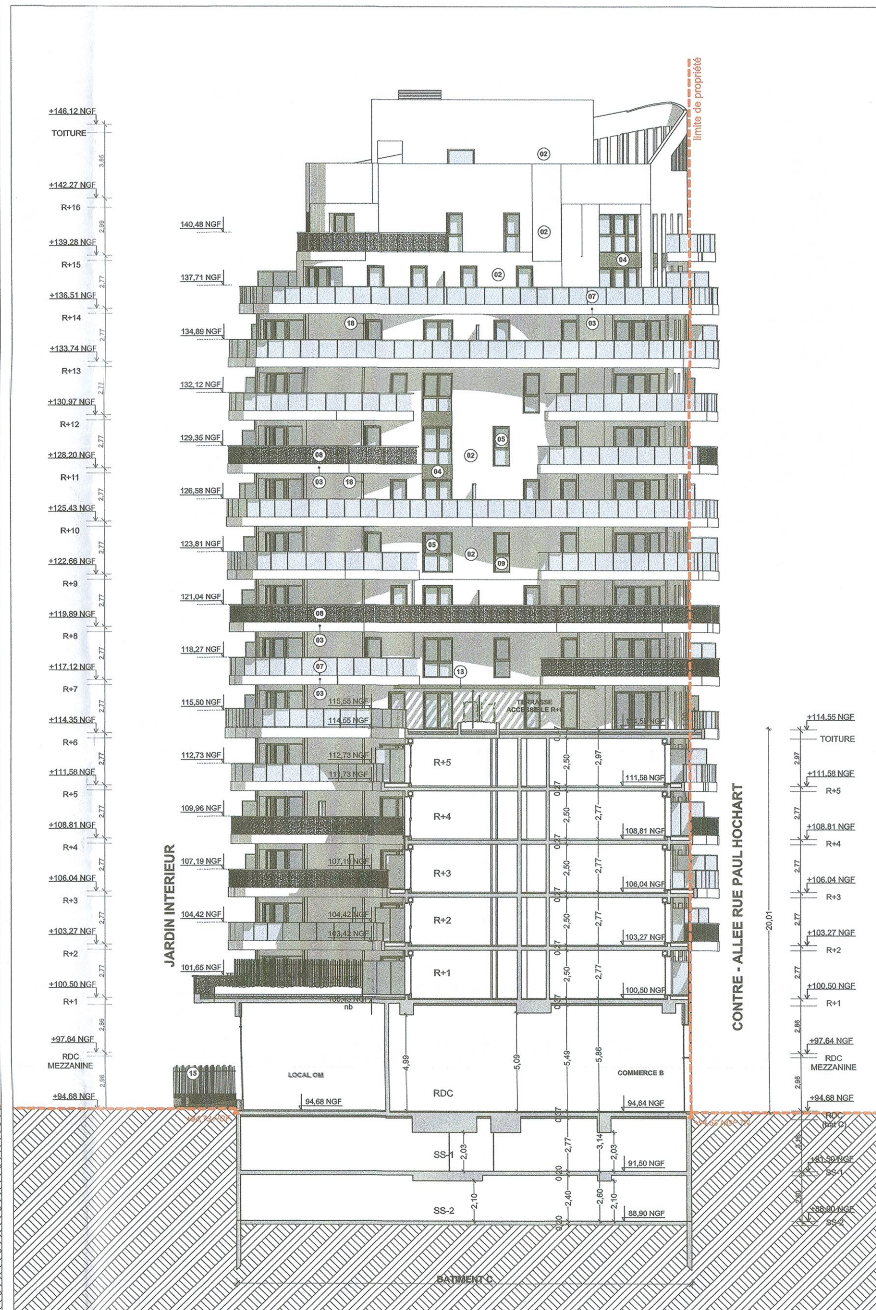
COUPE-FACADE CC
