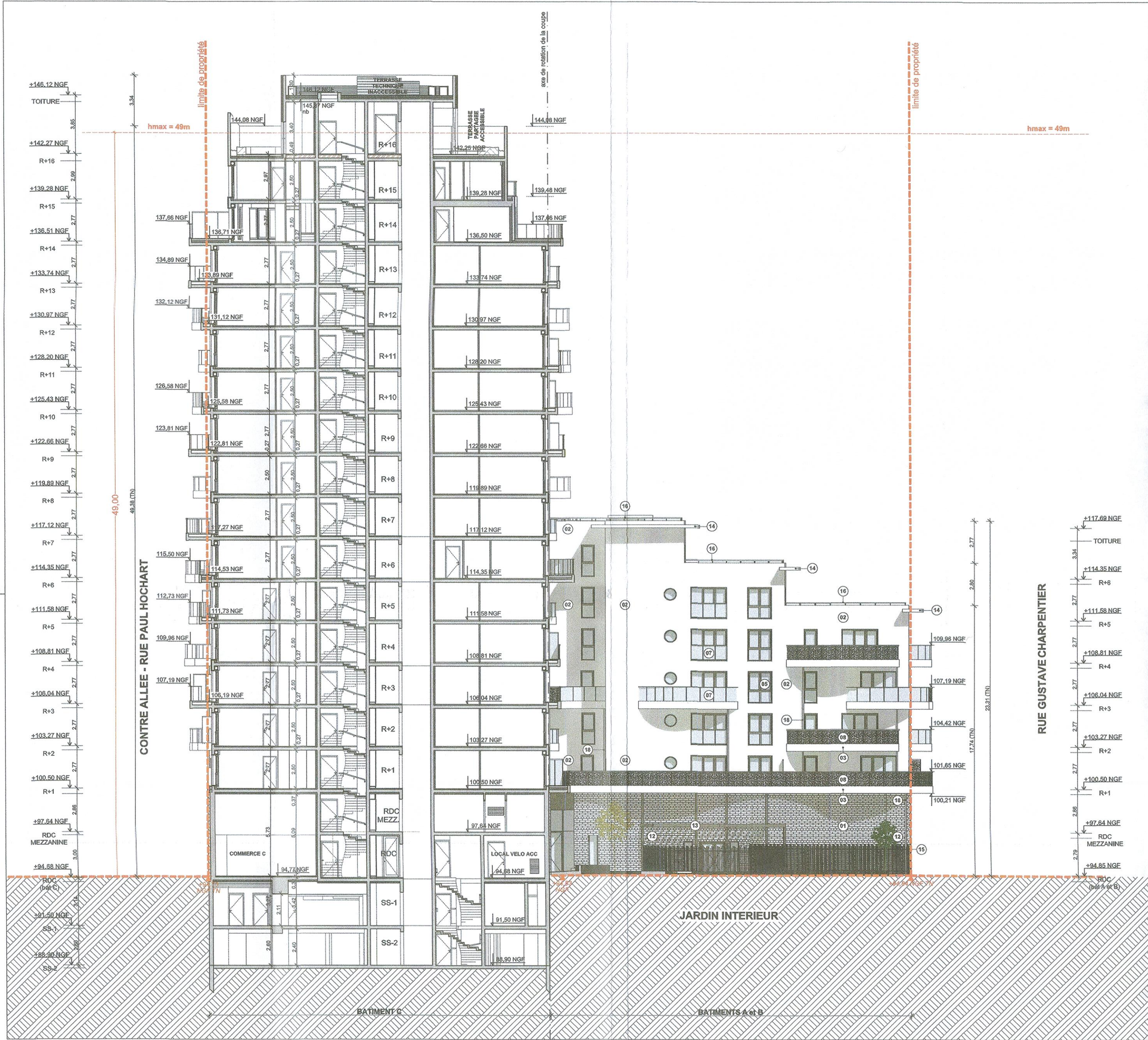
COUPE-FACADE AA
